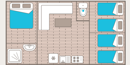
Dimensions : 8 x 4m - Terrasse : 6 x 2,50m
