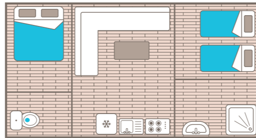
Dimensions : 7,80 x 3m - Terrasse : 4,50 x 2,50m
