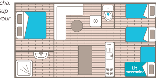
Dimensions : 9 x 4m - Terrasse : 6 x 3m
