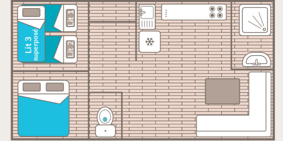
Dimensions : 5,40 x 4m - Terrasse : 4,50 x 2,50m
