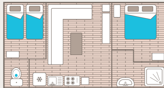
Dimensions : 7,30 x 4m - Terrasse : 4,50 x 2,50m
